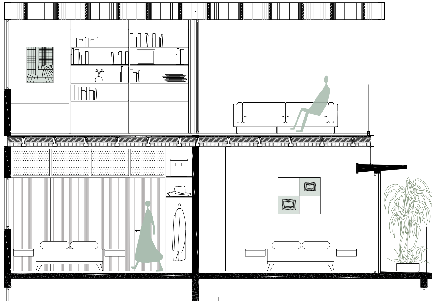
CORTE 3 - PH
